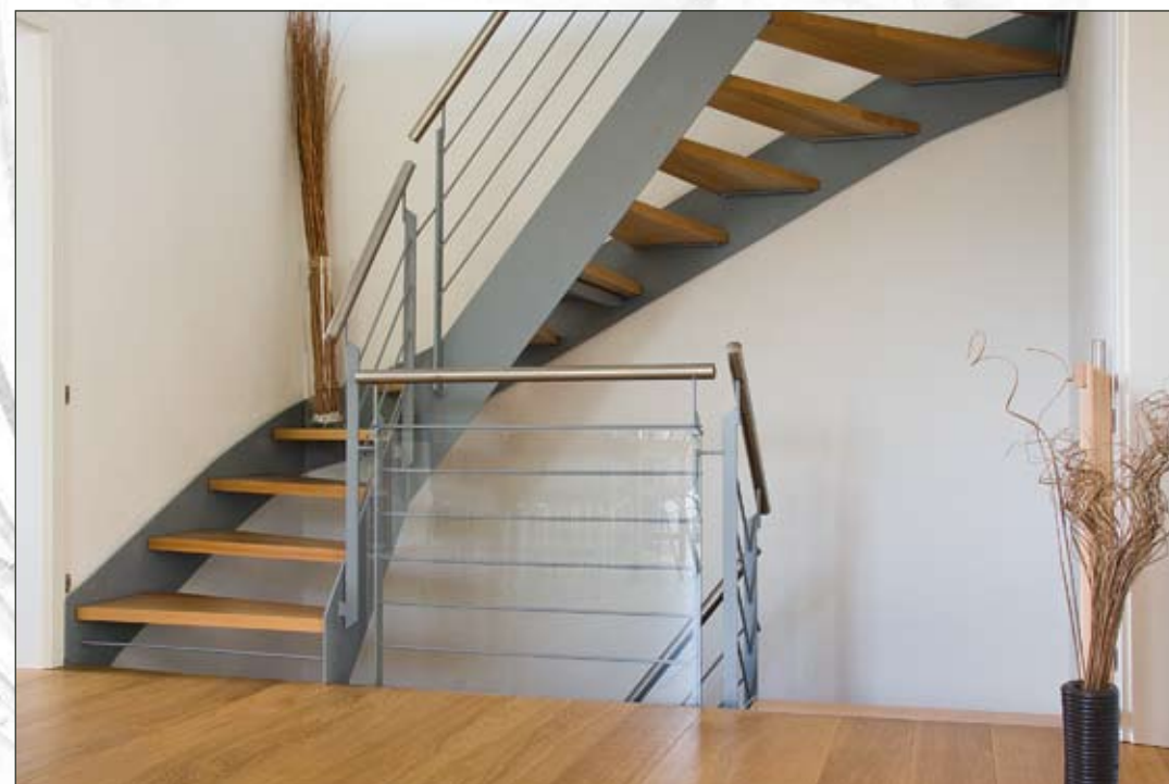
26 Flachstahlwangentreppe 2 x ¼-gewandelt mit horizontalen Stäben. Stufen in Buche, Edelstahlhandlauf.
